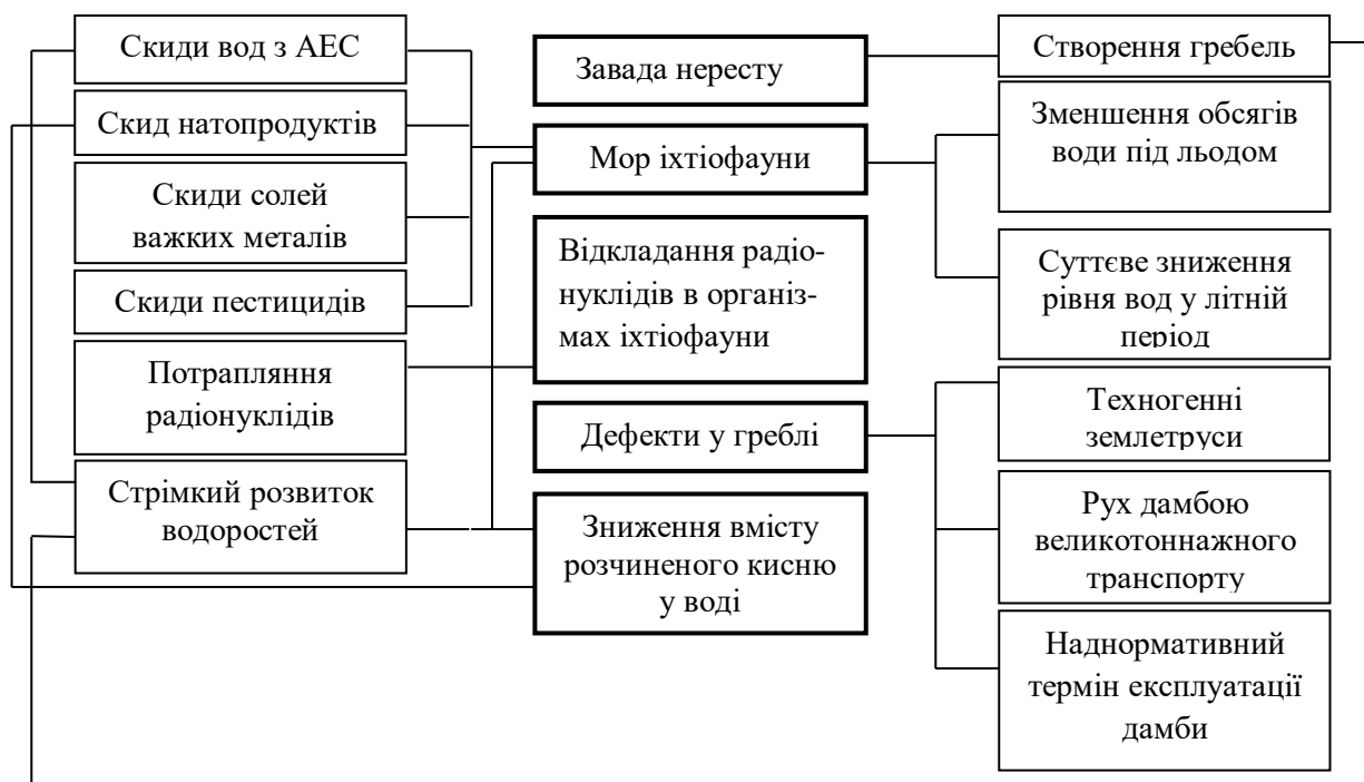
Рисунок 4.4 – Схема формування екологічної небезпеки в акваторіях Дніпровських водосховищ на території КСЕЗ
