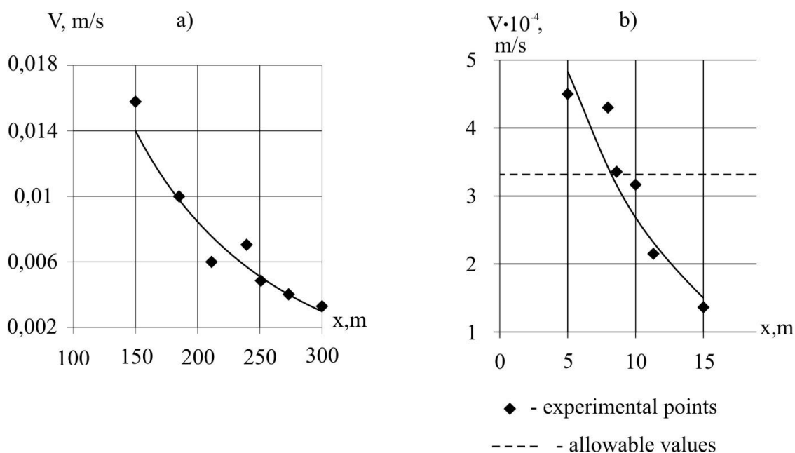
Рисунок 5.11 – Швидкість зміщення V на різних відстанях X від джерел ТЗ :
