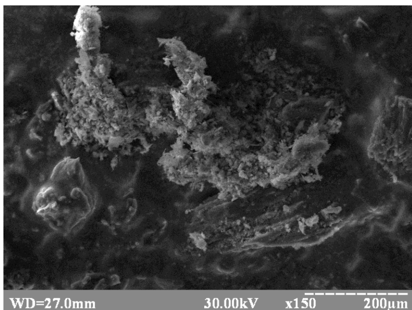
Рис.6.14. Електронно-мікроскопічні знімки поверхні гранульованих матеріалів: а) глауконіту з адсорбентом на основі соняшникового лушпиння; б) глауконіту з активованим вугіллям.
