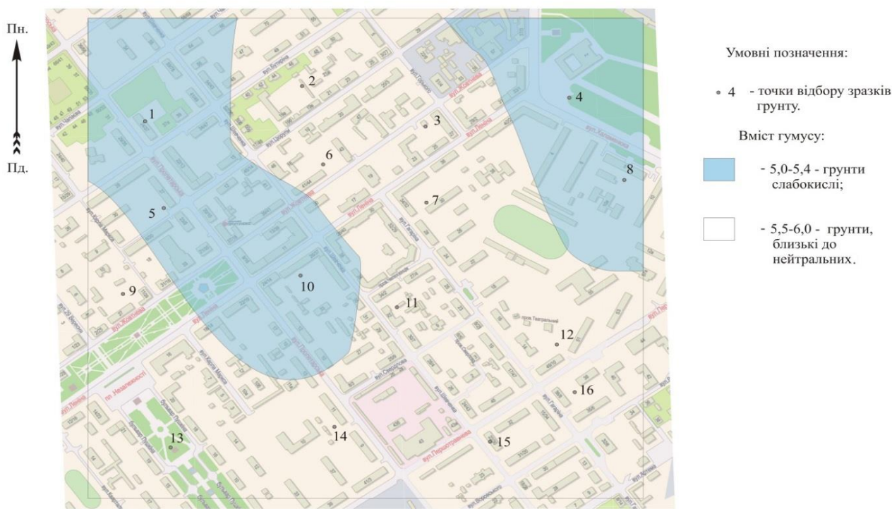
Рисунок 4.6 – Характеристика рН ґрунту у центральній частині КСЕЗ
