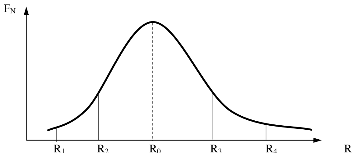
Рисунок 3.3 – Теоретична крива розподілу щільності проявів екологічної небезпеки F_N в СЕЗ залежно від її величини R ( R_1 – природний фон; R_2, R_3, R_4 – нижні рівні прийнятної, неприйнятної, катастрофічної небезпеки, відповідно; R_0 – середній для соціально-економічної зони рівень небезпеки)
