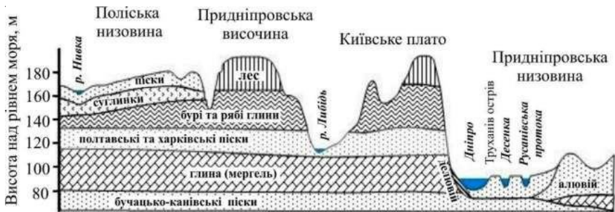
Рис. 5.3. Вертикальний геологічний розріз території м. Києва із Заходу на Схід
