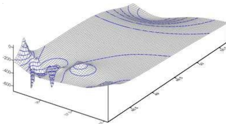
Рис. 3.4. Визначення теплового баричного поля поверхні Батиєвої гори м. Кісва у червні 2020 р. (А), листопаді 2021 р. (Б) та 3D-модель середнього теплового баричного поля (В). Значення ізоліній: 210, 200, 300, 350 – сумарне значення температурного нагрівання поверхні протягом року
