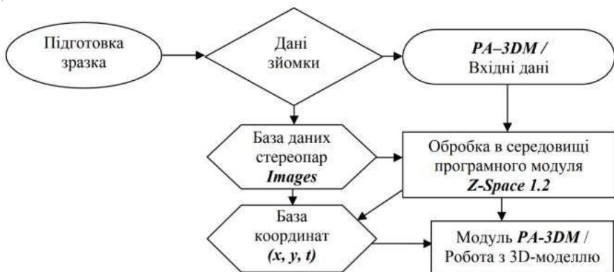
Рис. 3.2. Технологічний ланцюг отримання тримірної теплофізичної моделі
