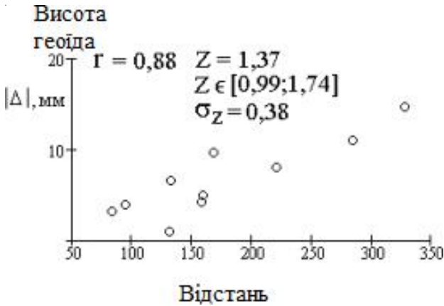
Рис. 5.45. Профіль висоти геоїда, отриманий методом GPS-нівелювання
